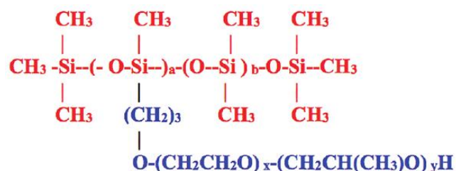
图 1. PEG/PPG 聚二甲基硅氧烷(3)。蓝色部分是水可溶部分，红色部分是硅油可溶部分
